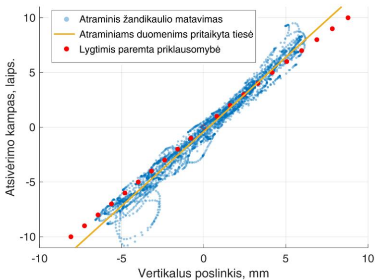
4.10 pav. Horizontalaus (šoninio) žandikaulio poslinkio ir šoninio pasisukimo kampo priklausomybės. Išmatuota ir apskaičiuota pasiūlytomis lygtimis. Koreliacijos koeficientas tarp atraminiu metodu įvertintų ir lygtimis apskaičiuotų priklausomybių tiesių yra 0,9996
