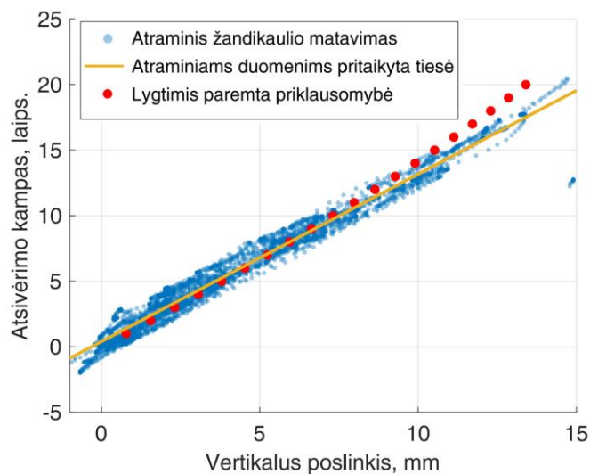
4.9 pav. Vertikalaus žandikaulio poslinkio ir atsivėrimo kampo priklausomybės. Išmatuota ir apskaičiuota pasiūlytomis lygtimis. Koreliacijos koeficientas tarp atraminiu metodu įvertintų ir lygtimis apskaičiuotų priklausomybių tiesių yra 0,9989
