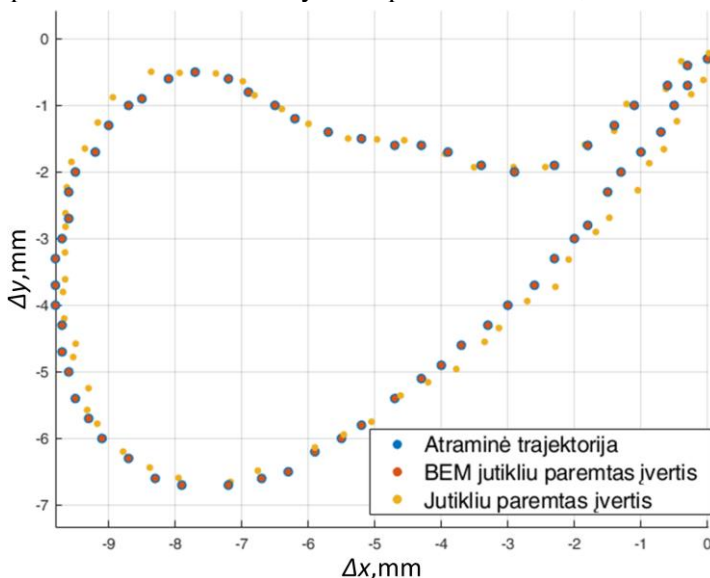
4.8 pav. Bandomoji trajektorija, nustatyta dviejų magnetometrų metodu su FML kompensavimu. Su teoriniais BEM duomenimis VKP = 0,05 \text{ mm} (raudona), o su eksperimentiniais „Elinta“ trimačio (3D) pozicionavimo sistema užfiksuotais duomenimis VKP = 0,28 \text{ mm} (geltona)
