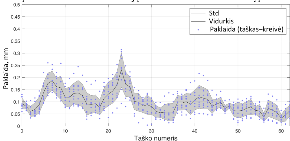
4.17 pav. Statinis 5-LL tyrimas. Lokalizacijos kiekvieno taško paklaidos ir Euklidinis atstumas (taškas-kreivė) per 10 kreivės matavimo iteracijų su vidurkiu ir standartiniu nuokrypiu
