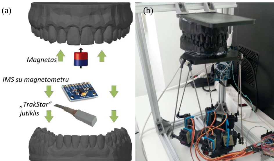
3.5 pav. Eksperimento schema dinaminiam lokalizacijos tyrimui su dinaminio okliuzijos nustatymu (a), panaudojant Stiuarto platformą (b)
