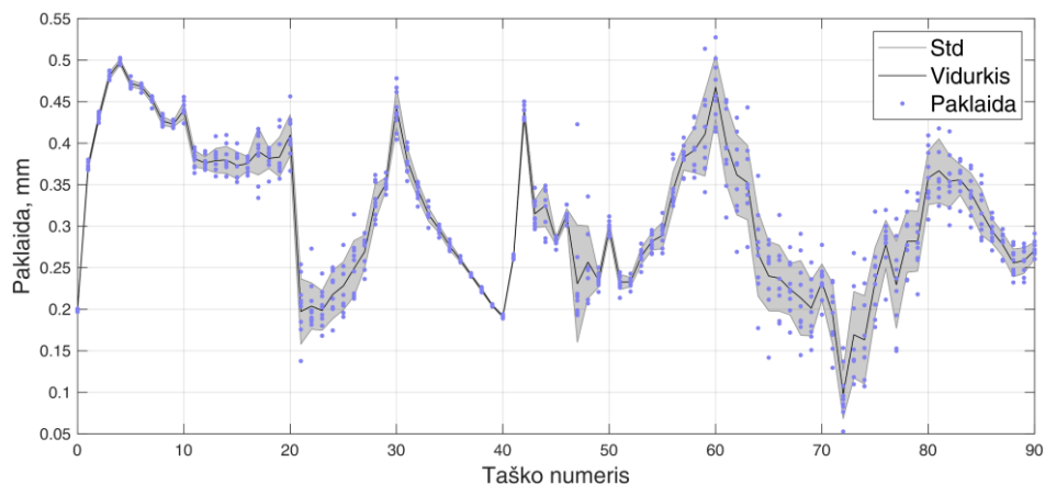
4.2 pav. Kiekvieno taško lokalizacijos paklaida per 10 kubinės bandomosios trajektorijos matavimo iteracijų su vidurkiu ir standartiniu nuokrypiu
