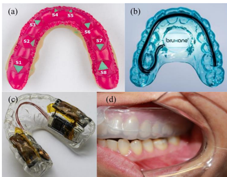
1.2 pav. Okliuzinės kapos bruksizmo diagnostikai: (a) nusitrinančios kapos pusiau automatiniam vertinimui skenuojant [24]; (b) „Bruxane“ kapos su integruotais slėgio jutikliais [25]; (c) kapa su integruotais pjezorezistiviais slėgio jutikliais [5]; (d) kapa su optinio pluošto slėgio jutikliais [26]
